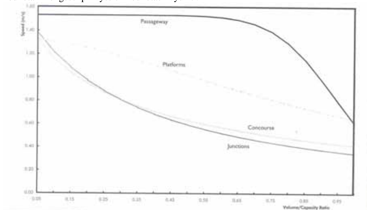
Obr. 2 Rychlost pohybu pěších ve vztahu ke kapacitě
